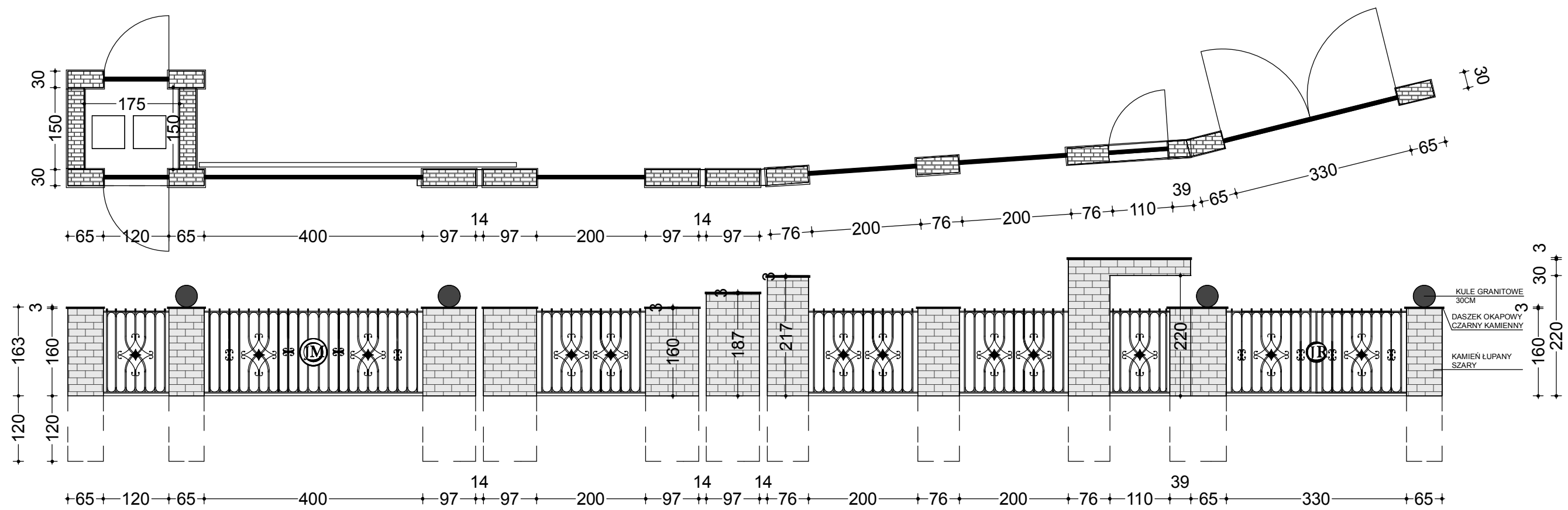
PROJEKT OGRODZENIA RZUT SKALA 1:50
